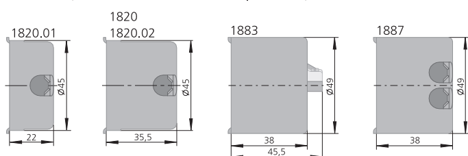
Scatole di protezione contro i contatti | Contact protection boxes
