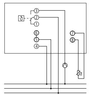
RAMSES 832 top2
