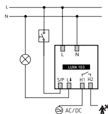
LUXA 103 S360-100
