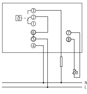
RAMSES 832 top2
