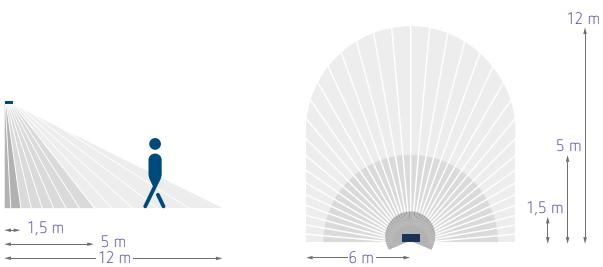
theLuxa S180
