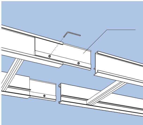
Montage Steigeleitern Abstand Wandhalter \leq 2 m
