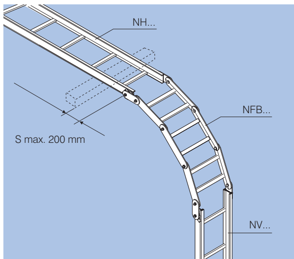
Gelenkleiter vertikal
