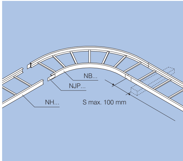
90° Bogen waagrecht
