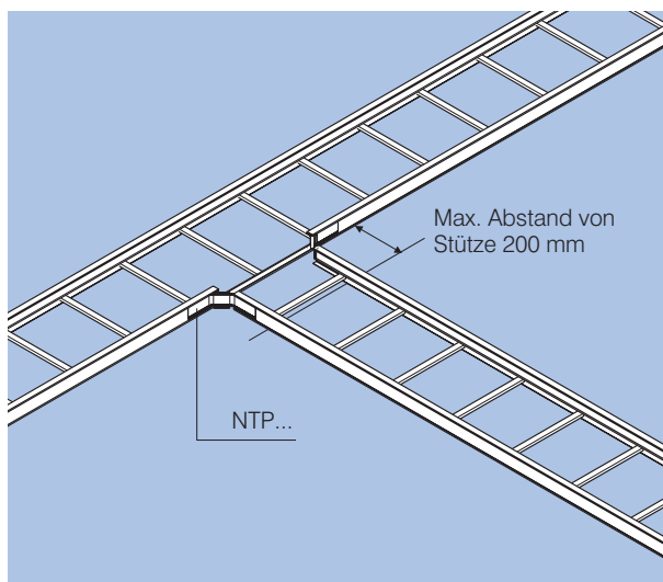
Winkelverbinder
