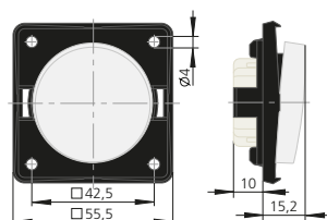
Interruttore/pulsante a bilanciere Switch/Push button
