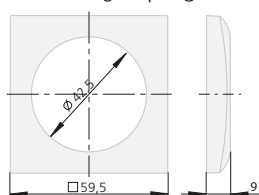
Cornici singola | Single frame
