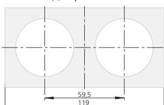
Cornici doppia | Double frame
