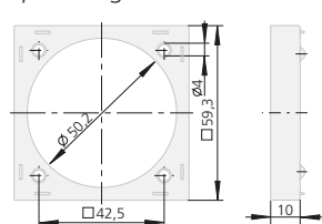
Distanziatore Spacer ring
