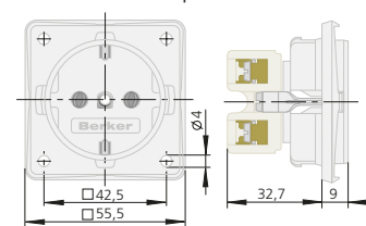
Presa da incasso | Built-in socket
