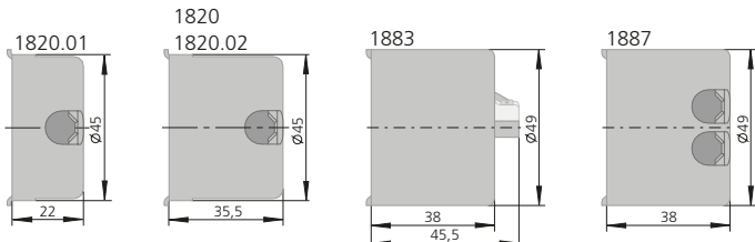
Scatole di protezione contro i contatti | Contact protection boxes
