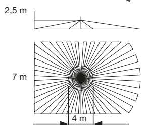
zona "P" di massima rilevazione area "P" of maximum detection
