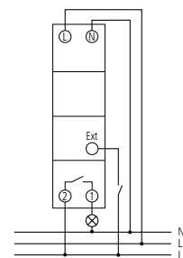
SELEKTA 175 top2
