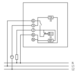
RAMSES 705
