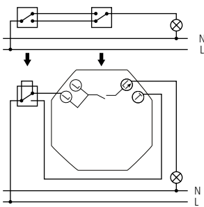
LUXA 103-200 T
