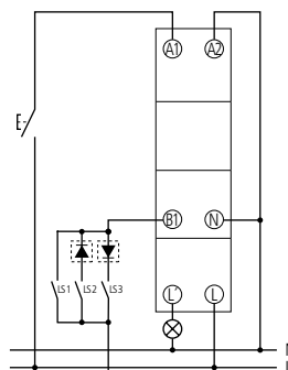
DIMAX 534 plus
