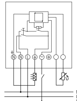
RAMSES 751 RA
