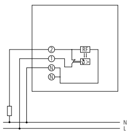
RAMSES 701
